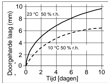
Schema 1: Uithardingsnelheid voor Sikaflex®-298 FC
